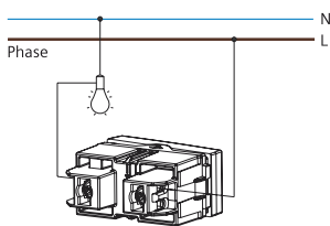
สวิตช์ทางเดียว
