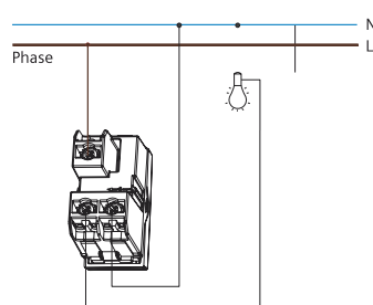
สวิตช์ทางเดียว (แบบเปิดมีไฟ)
